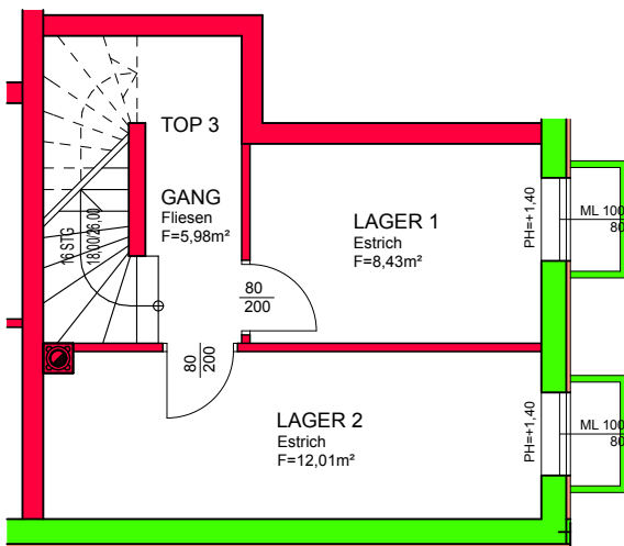
Kellergeschoss M 1:100
