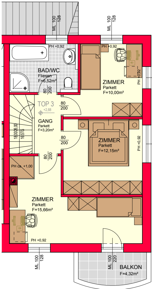
Obergeschoss M 1:100
